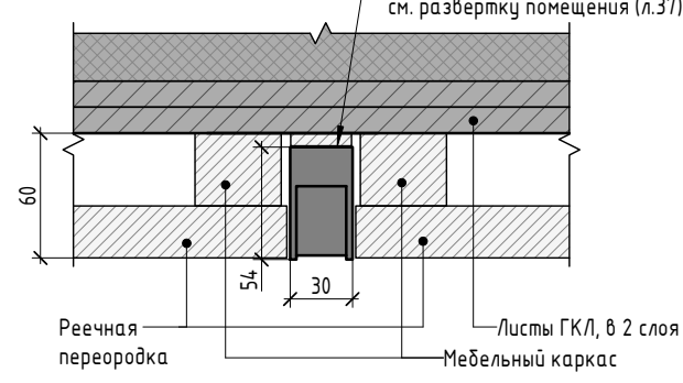
Узел 2
